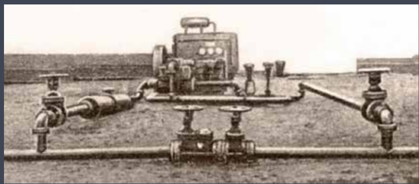
ПОЛЕВАЯ НАСОСНАЯ УСТАНОВКА
